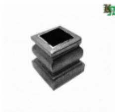
Вставка в балясину, арт. 103.20 40x40мм, на кв.20x20мм Вес: 0.13 кг Цена: 75 руб.
