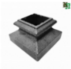
Вставка в балясину, арт. 277.30 70x43мм, на кв.30x30мм Вес: 0.45 кг Цена: 150 руб.
