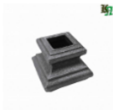
Вставка в балясину, арт. 1376.14 28x37мм, на кв.14x14мм Вес: 0.17 кг Цена: 28,90 руб.
